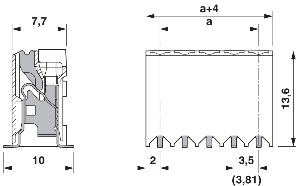
尺寸图
