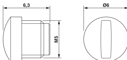
Maßzeichnung
