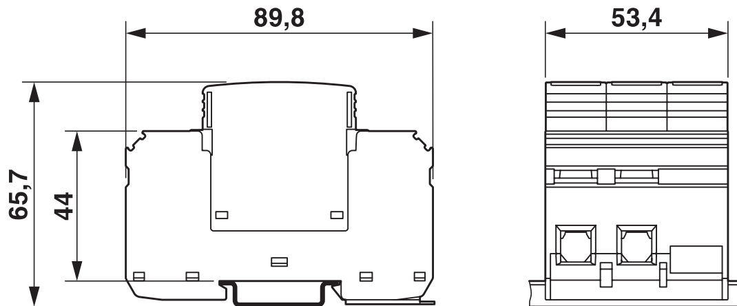
尺寸图
