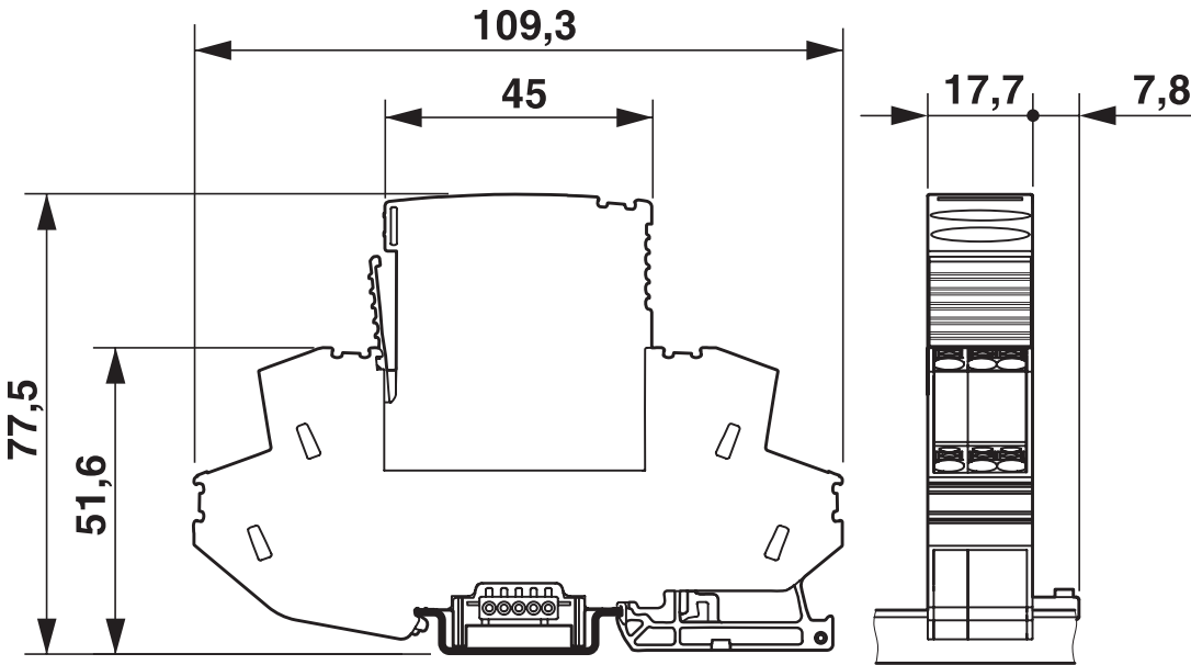
尺寸图
