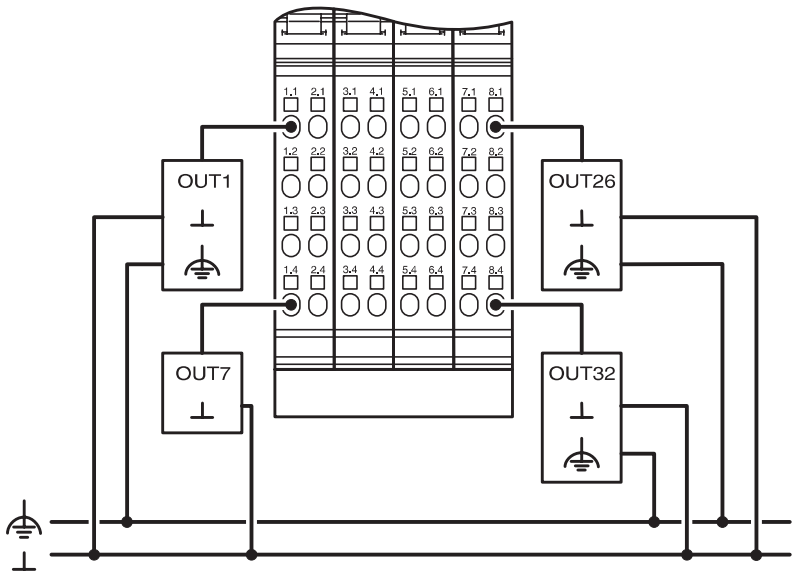
接线图
