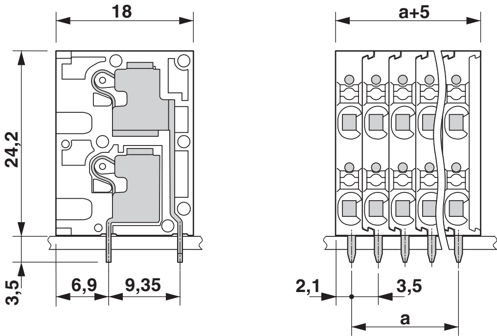
尺寸图
