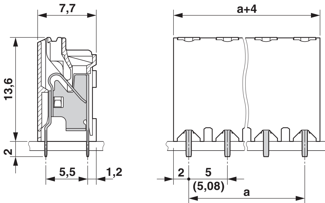
尺寸图
