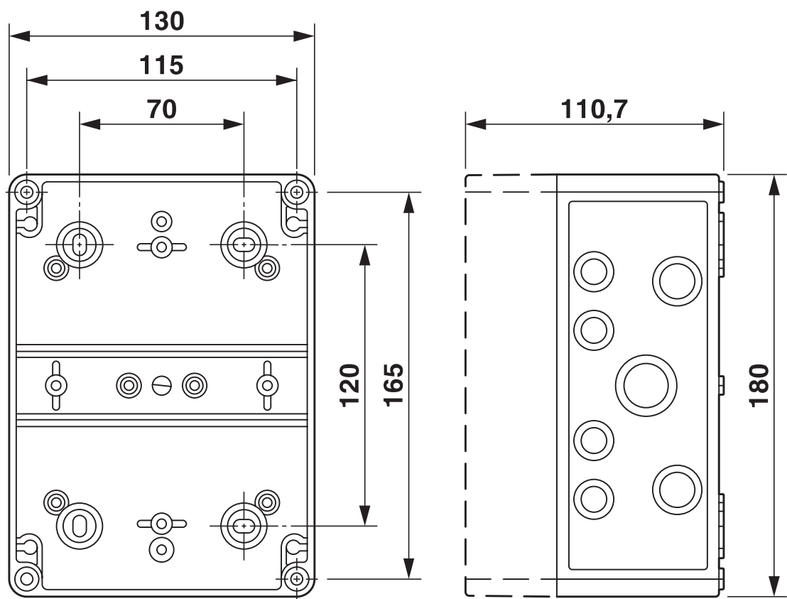
尺寸图
