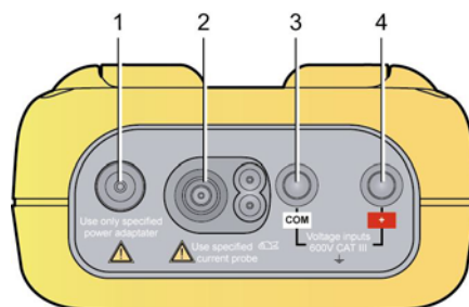
Abbildung 2: Die im oberen Teil vorhandenen Anschlüsse.
