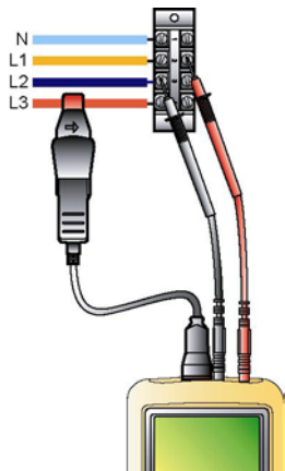
Abbildung 75: Symmetrischer dreiphasiger Anschluss. 006
