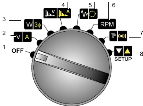
Abbildung 6: Ansicht der ausgehend vom Drehschalter verfügbaren Modi.
