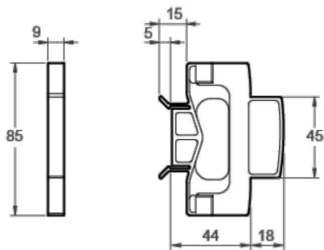
尺寸(mm)
