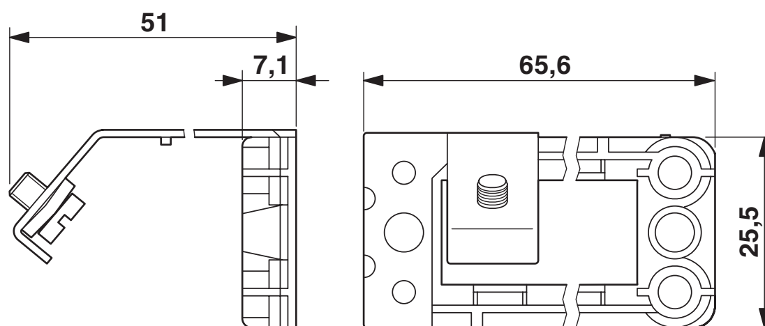
尺寸图
