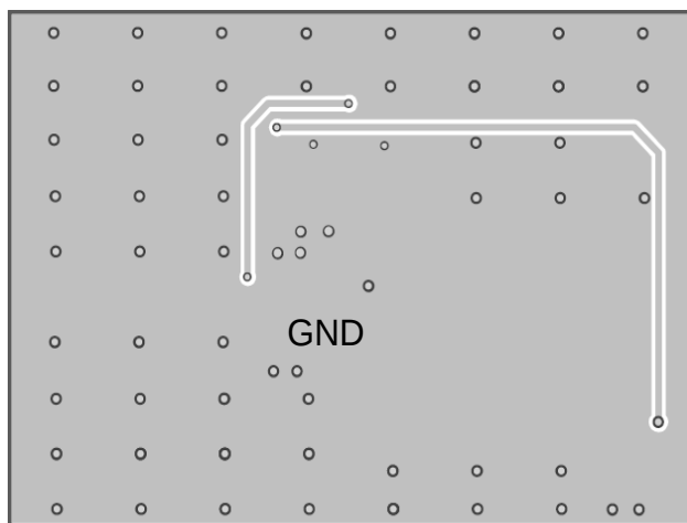
Bottom Layer
