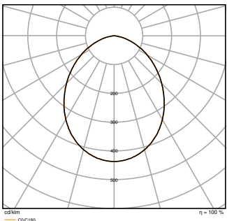
DL CMFT ZB D100 P 13W 930 OP WT
