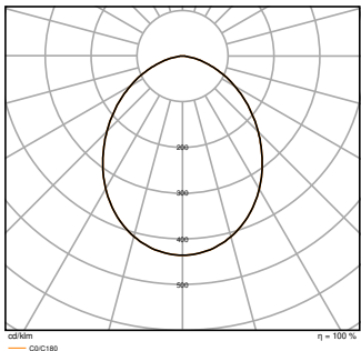
DL CMFT ZB D100 P 13W 940 OP WT
