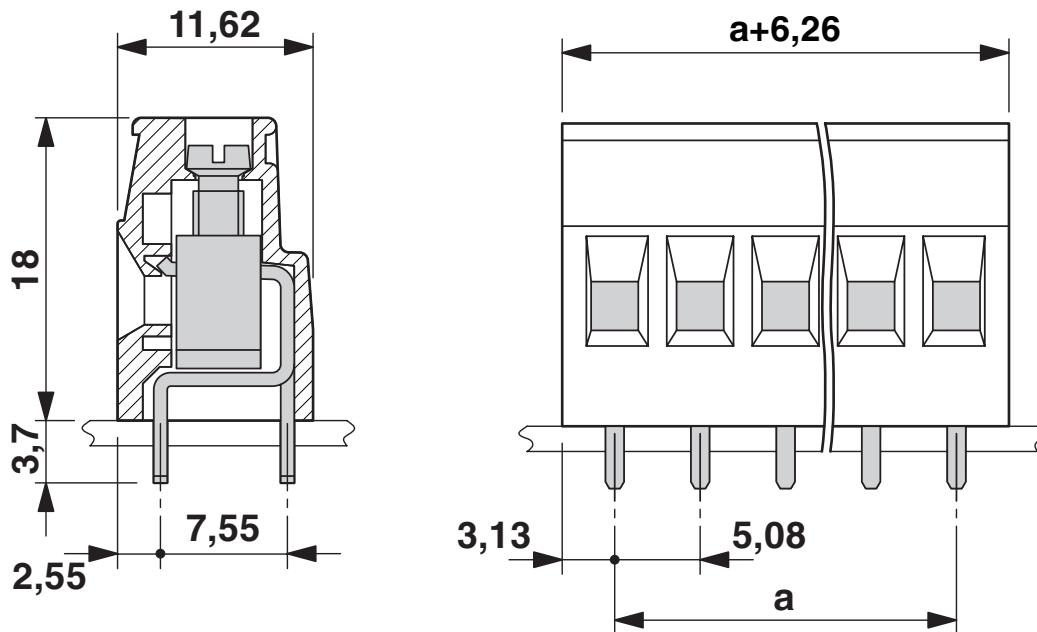
尺寸图
