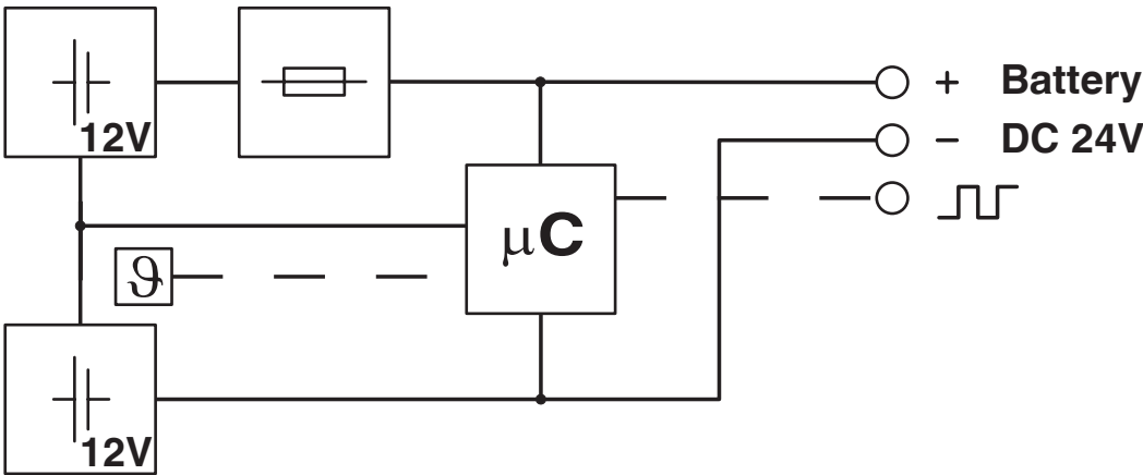
结构框图
